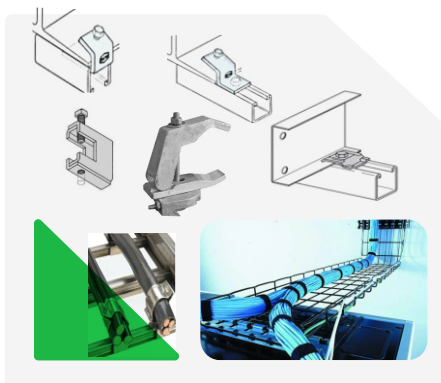
Bandeja Portacable
